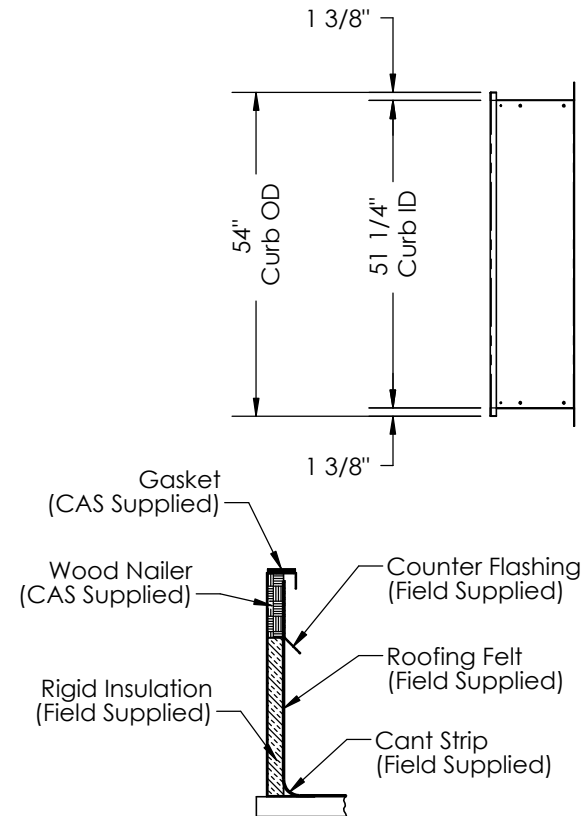
TYP Cross Section
